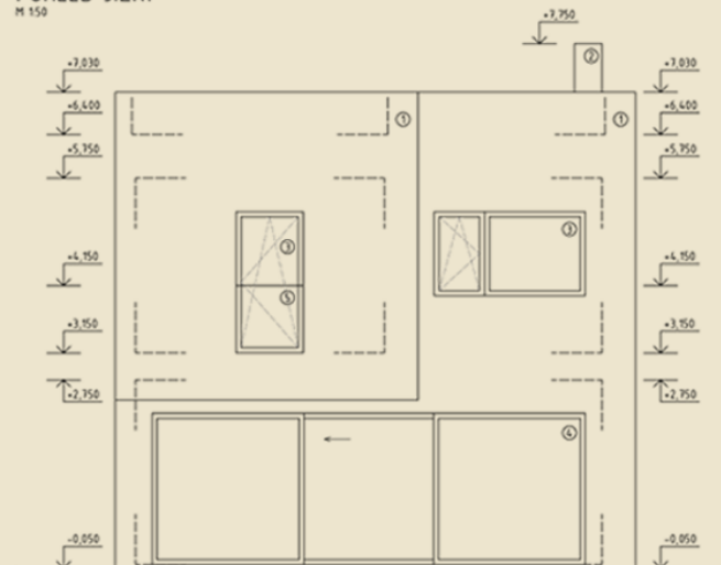
POHLED JIŽNÍ M 1:50
