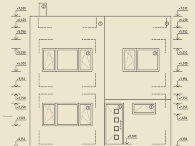
POHLED SEVERNÍ M 1:50
