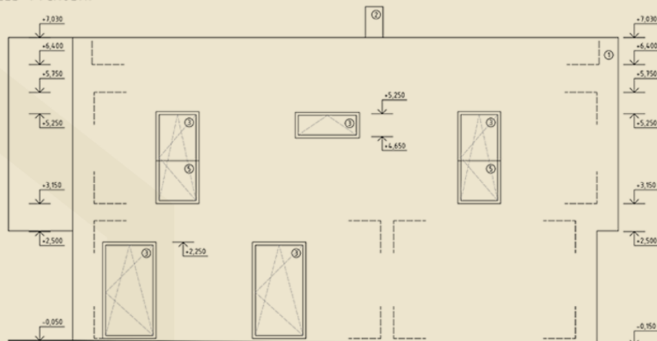
POHLED VÝCHODNÍ M 1:50
